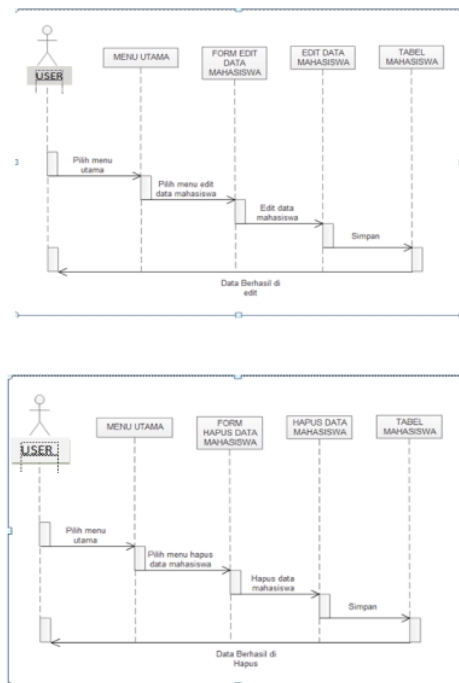
Gambar 4. Sequence Diagram Aplikasi Data Mahasiswa
